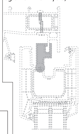
Widok Y2 (Zamontowany ogranicznik skrzydła)
