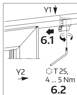
Widok Y1 (bez szyny prowadzącej)
