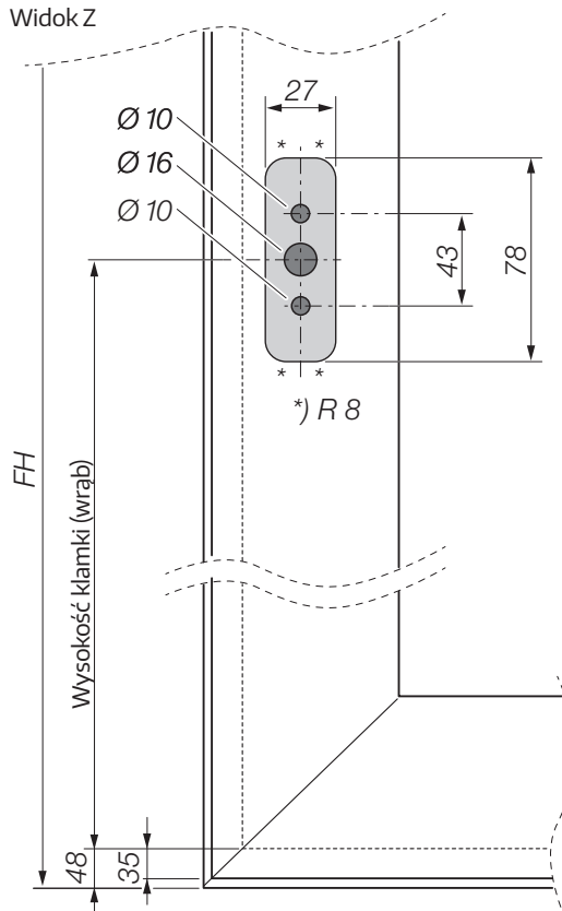
Widok Z
