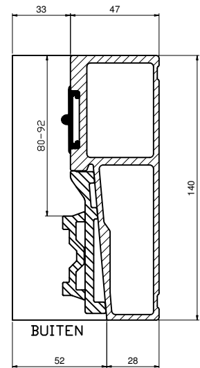
uitvoering rechts lage rail
