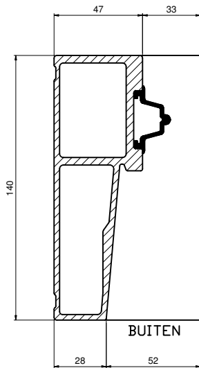
uitvoering rechts hoge rail
